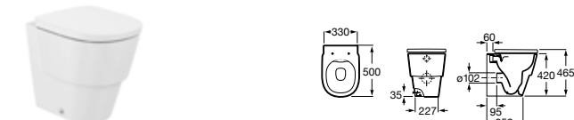
Inodoro de tanque alto o empotrable adosado a pared 500 mm de longitud Blanco Colores mate
