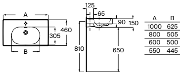
Lavabo mural con juego de fijación
