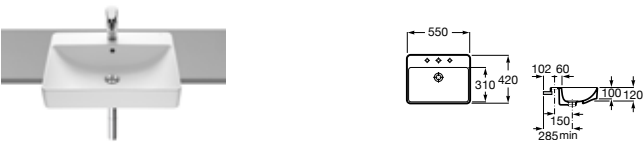
Lavabo semiempotrar con juego de fijación Blanco Colores mate 550 x 420 A32753S..0 € 282,00 € 337,00
