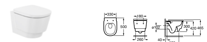
Inodoro suspendido 500 mm de longitud Blanco Colores mate
