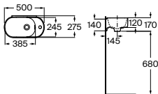
Lavabo asimétrico mural compacto con juego de fijación
