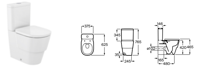
Inodoro de tanque bajo adosado a pared 625 mm de longitud Blanco Colores mate
