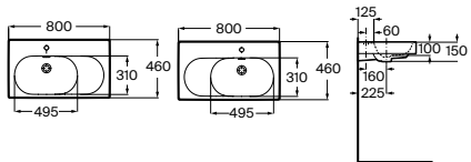
Lavabo mural asimétrico con juego de fijación
